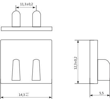
Заглушка на 3-полюсную шину
